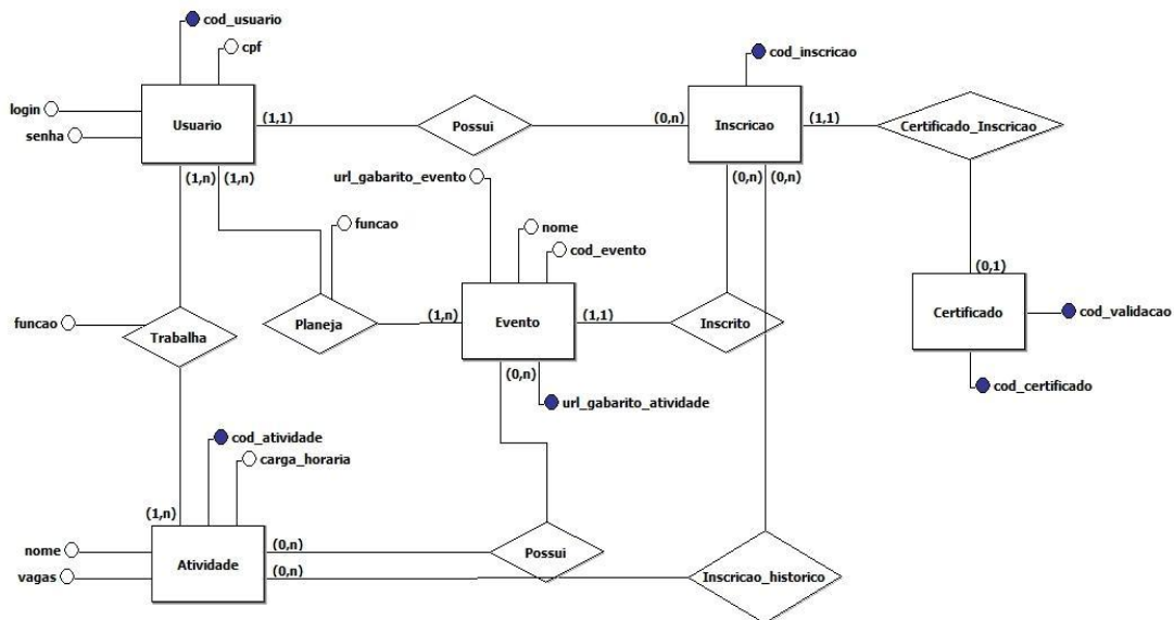
Figura 4. Modelo conceitual do banco de dados do e-Vent-Br.
